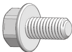
12 Boulon à épaulement M8 – 1,25 X 16
