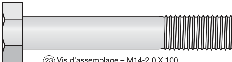
(23) Vis d'assemblage – M14-2,0 X 100
