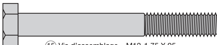
(15) Vis d'assemblage – M12-1,75 X 95
